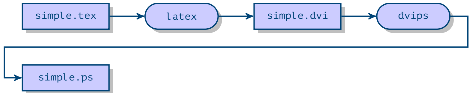
Рис. 4: создание PostScript-файла
