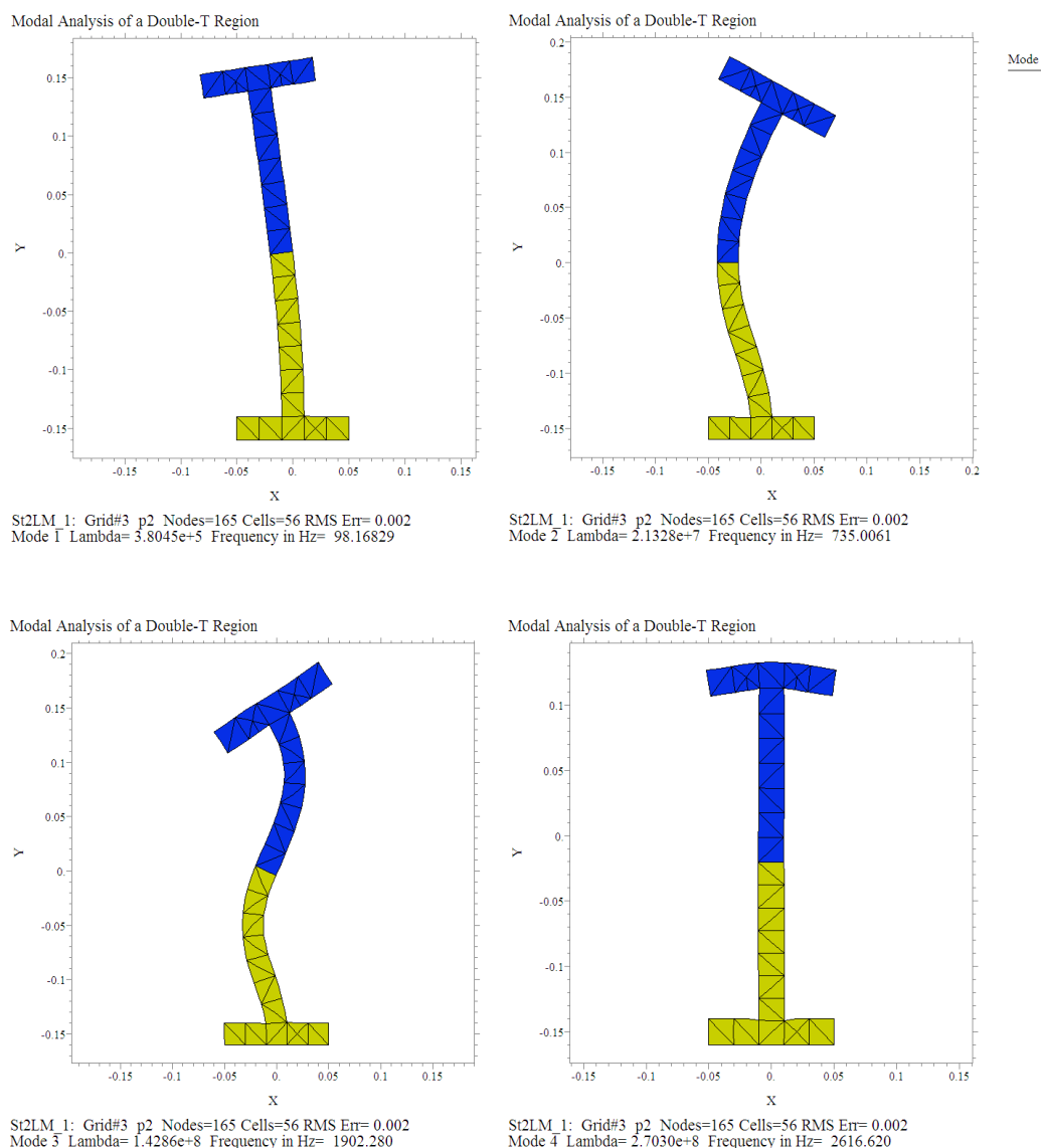
Рис. 4 Собственные формы колебаний (FlexPDE)
