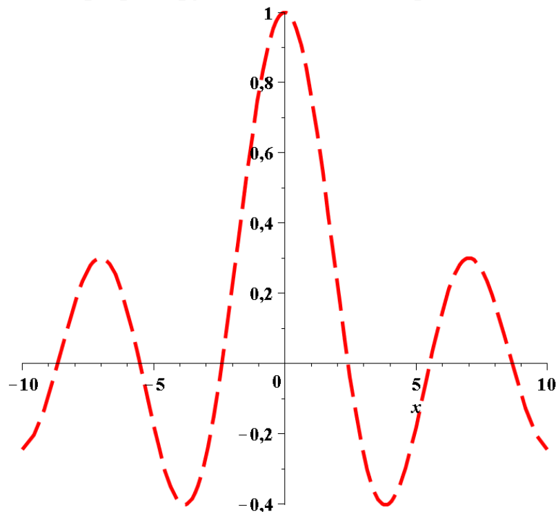
График функции Бесселя при n=0
