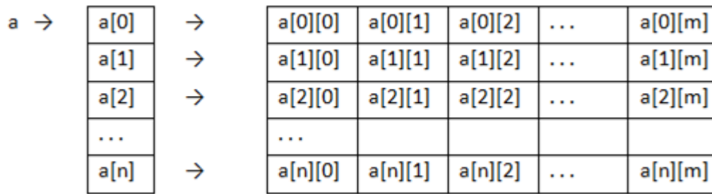
Рис. 2.1. Организация двумерного массива в динамической памяти
