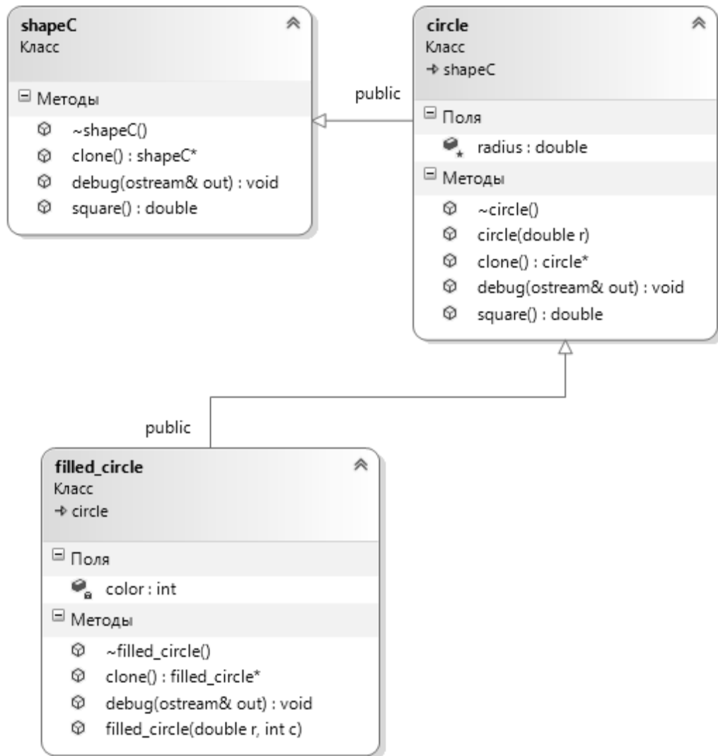
Рис. 6.5. UML диаграмма классов к примеру 87
