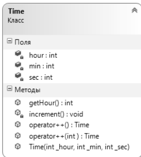
Рис. 5.2. UML диаграмма класса Time
