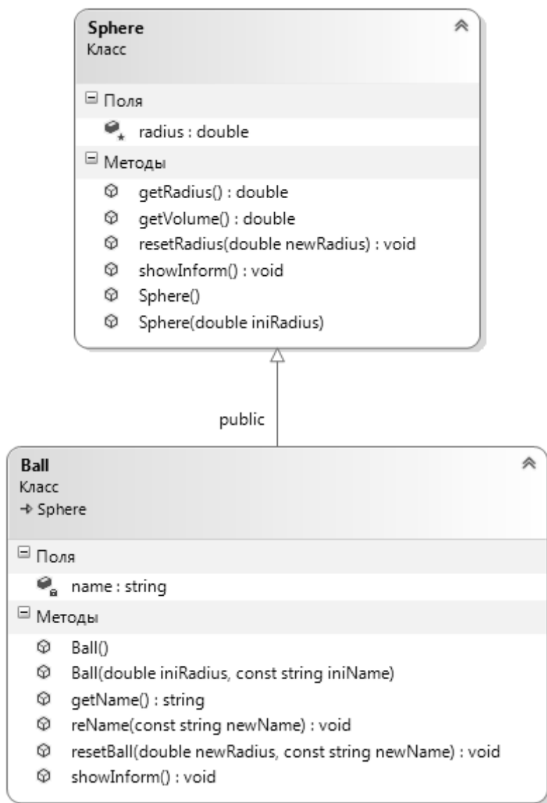
Рис. 6.1. UML диаграмма иерархии классов Sphere – Ball
