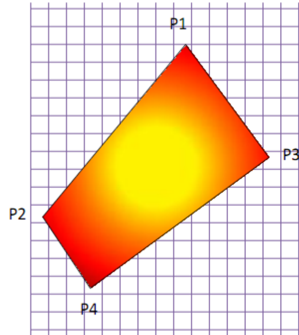
Фонг
