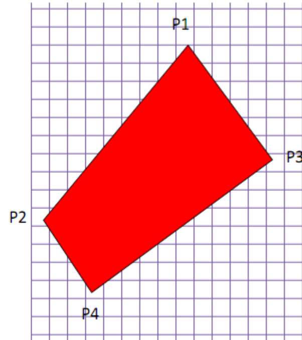
Гуро
